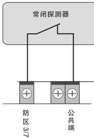
2) 不带电阻的常闭接法:
