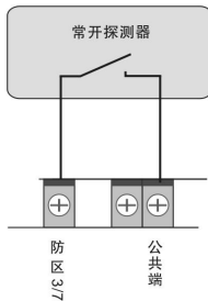
1) 不带电阻的常开接法:
