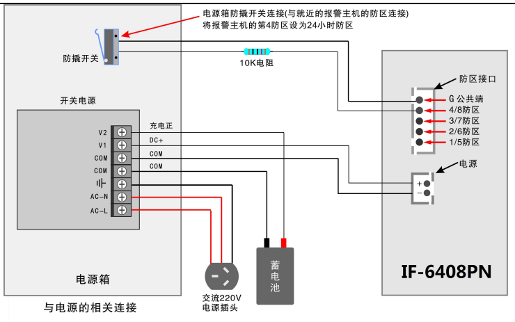
IF-6408PN 与电源箱的连接
