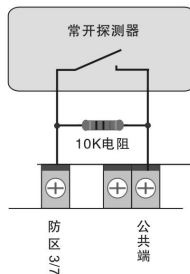
3) 带 1 个电阻的常开接法:
